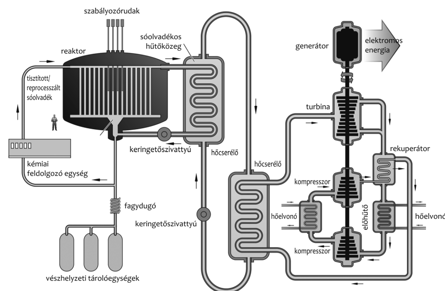
9. ábra • Sóolvadékos reaktor (URL)
