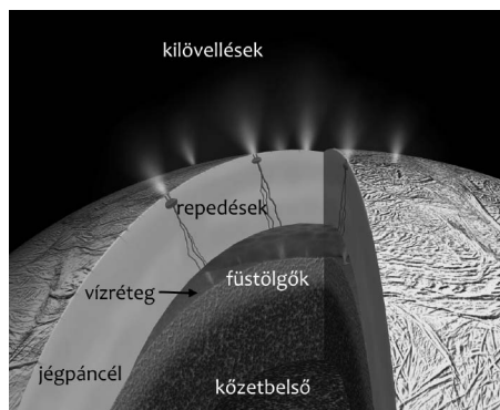
4. ábra • Az Enceladus hold feltételezett belső szerkezete: a mélyebben lévő szilikátos anyag a mélységi vízzel kölcsönhatásba lép, majd a víz a repedéseken keresztül részben eltávozik a világűr felé (NASA, JPL).
