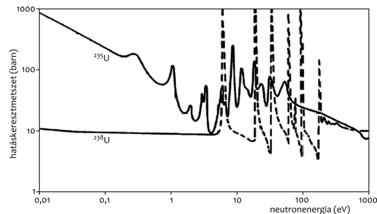
1. ábra • Az uránizotópok hatáskeresztmetszetének energiatartomány szerinti függése
