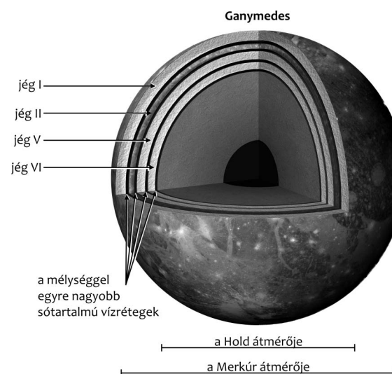
3. ábra • Vázlat a Ganymedes lehetséges belső szerkezetéről: eltérő mélységben több, különböző kristályszerkezetű jég réteg is lehet, amelyek között az oldott sók miatt cseppfolyós halmazállapotú vizes oldatok akár további rétegeket alkotnak (NASA, JPL)
