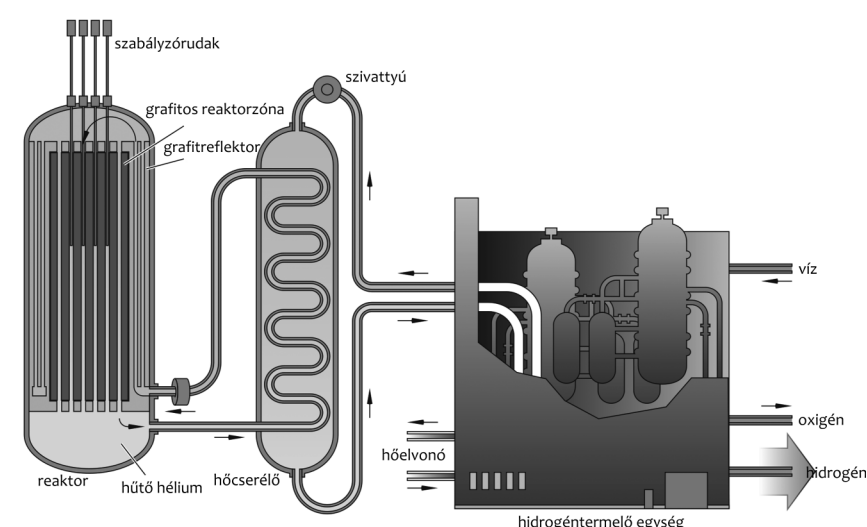
10. ábra • Gázhűtésű magas hőmérsékletű gyorsreaktor
