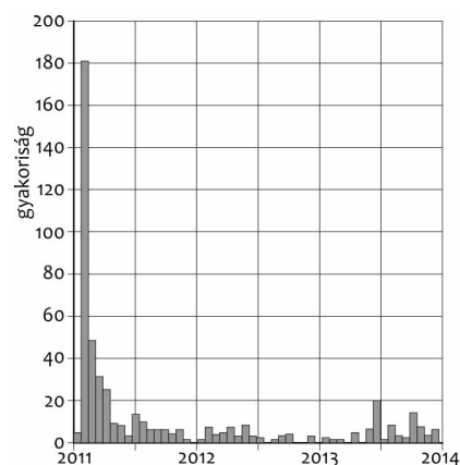
3. ábra • A Vértesszőlős térségében az elmúlt 3 évben kipattant földrengések időbeli története. A 2013 közepén megemelkedett rengésszám Bodajk és Mór között július első két napján kipattant 18 kisebb rengésnek köszönhető. Ezek már nem tekinthetők oroszslányi utórengéseknek.
