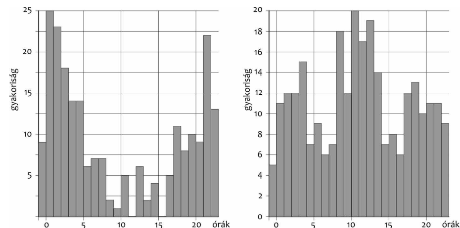
4. ábra • A földrengések napi eloszlása: balra az M<0,2 , jobbra az M>0,2 méretű földrengésekre
