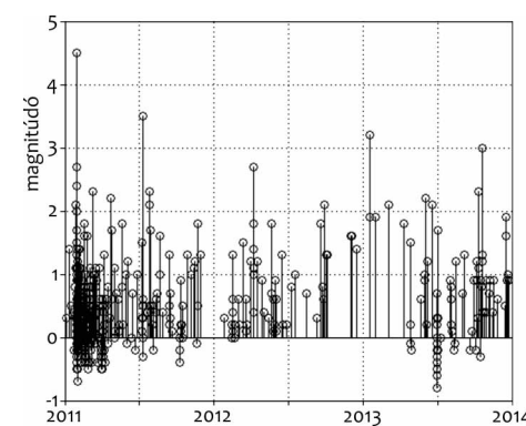
5. ábra • Az utórengések magnitúdótörténete. Látható, hogy az ideiglenes állomásoknak köszönhetően nagyon sok negatív magnitúdójú eseményt sikerült meghatározni közvetlenül a főrengés utáni hónapokban.
