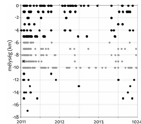
6. ábra • A földrengések mélység szerinti eloszlása. Az oroszslányi M=4,5 rengés 9 km mélyen keletkezett, amit X jelöl
