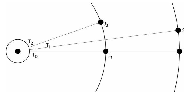
4. ábra • Az ilyen oszcillációk miért gyakoribbak a Szaturnusznál, mint a Jupiternél? Ha a Föld egyszerre ( T_0 ) előzi le a két bolygót ( J_1 és S_1 ) – vagyis azok egyszerre írnak le egy hurkot –, akkor egy földi keringés eltelte után a Föld először ( T_1 ) a Szaturnuszt ( S_2 ) éri utol ismét, és csak később ( T_2 ) a Jupitert ( J_2 ).
