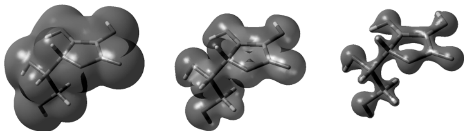
2. ábra • A C-vitamin molekulájának modellje az azonos elektronsűrűség-értékeket (bal oldalon: 0,004, középen: 0,04, jobb oldalon: 0,2) összekötő burkolófelület alapján. Feltüntetettük az atommagokat összekötő vonalak alkotta molekulavázát is.
