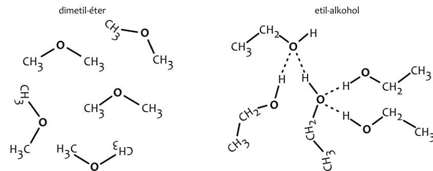
1. ábra • Míg az etanol hidrogén-hidakon keresztül (szaggatott vonalak) asszociátumok képzésére hajlamos, megemelve ezzel a folyadék forráspontját, addig a dimetil-éter ugyanilyen hálózatok kialakítására alkalmatlan.
