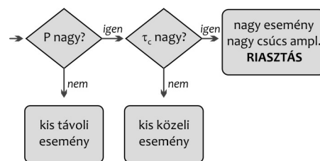
6. ábra • Földrengés-megfigyelő és -riasztó rendszer működésének folyamatábrája
