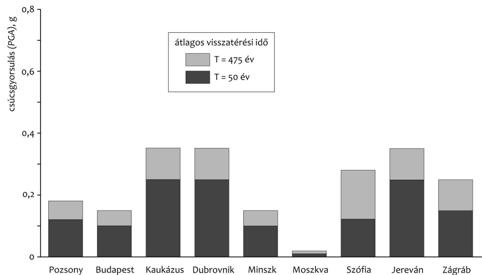
4. ábra • Közepes földrengés-visszatérési időintervallumok ( T=475 év és T=50 év) alapján számított PGA-értékek a világ különböző részein g -ben ( g=981 \text{ cm}\cdot\text{s}^{-2} )
